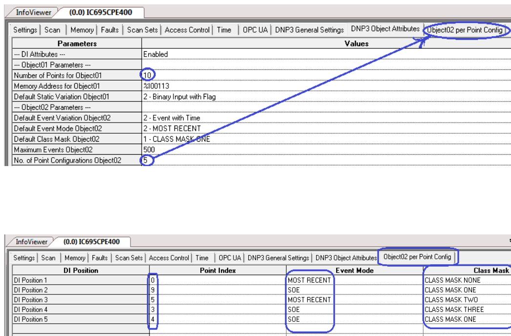
Figure 19: DI Attributes - Per-Point Configuration Parameters
