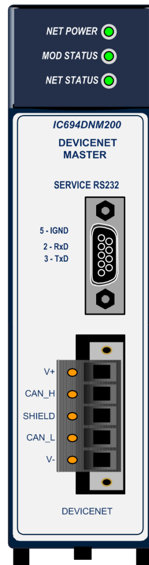
Figure 382: IC694DNM200
