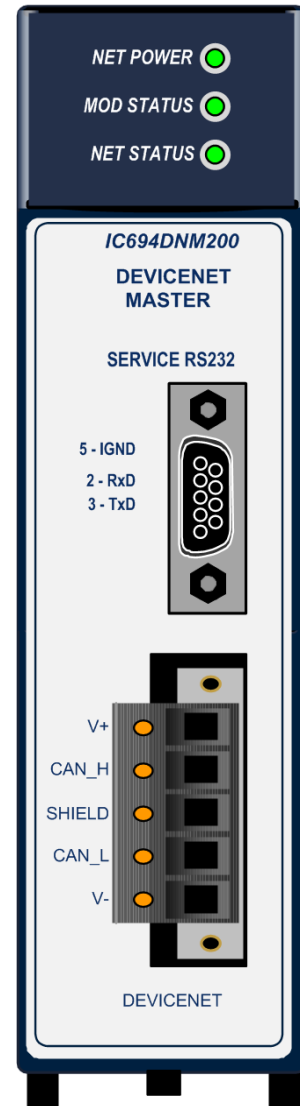
Figure 382: IC694DNM200
